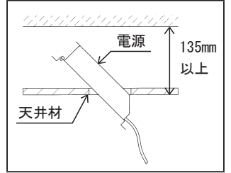
図1 埋込深さ
