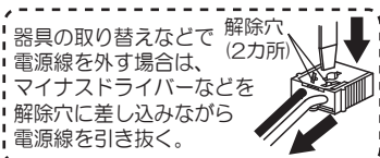
端子台
