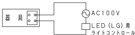
結線図
