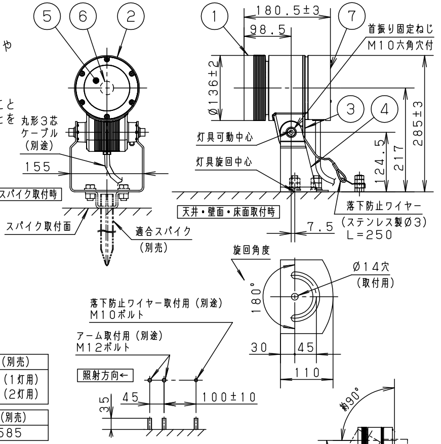
ボルト固定時の取付用ボルト配置図
