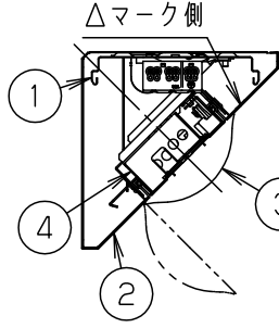
断面詳細図
