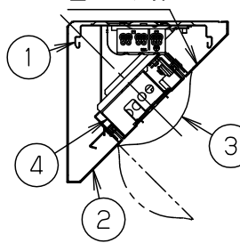
断面詳細図
