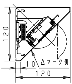
断面詳細図
