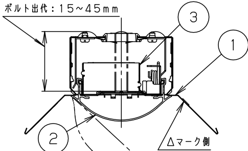
断面詳細図
