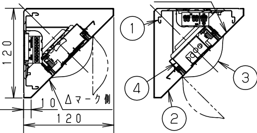
断面詳細図
