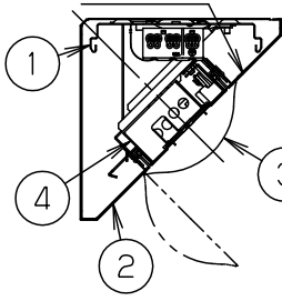
断面詳細図
