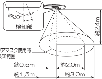
検知部を約20° 傾けた場合
