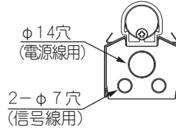
<器具端面図>
