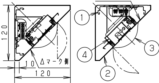
断面詳細図
