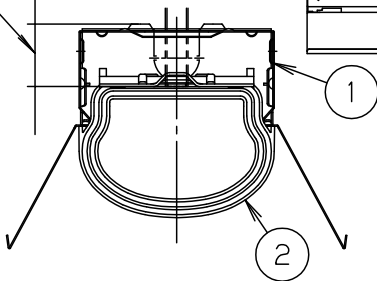
断面詳細図
