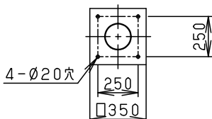
取付寸法図
