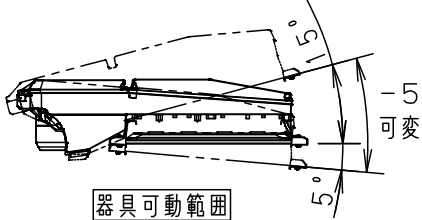
器具可動範囲
