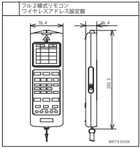
WRT9500K.DXF
