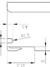
D部詳細図
