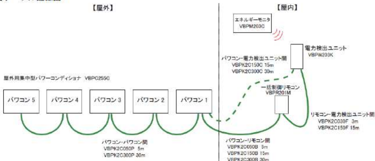
通信ケーブル配線図
