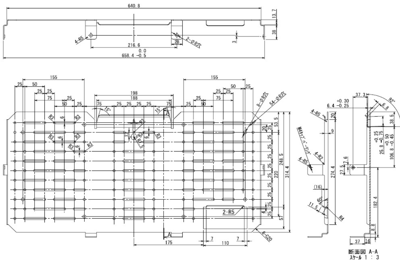
口外形寸法図
