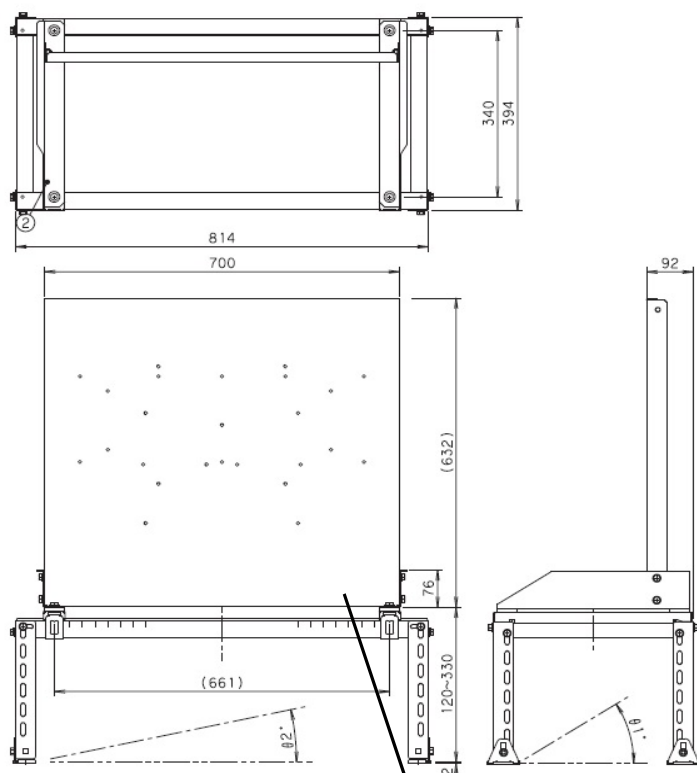
□外形寸法図
